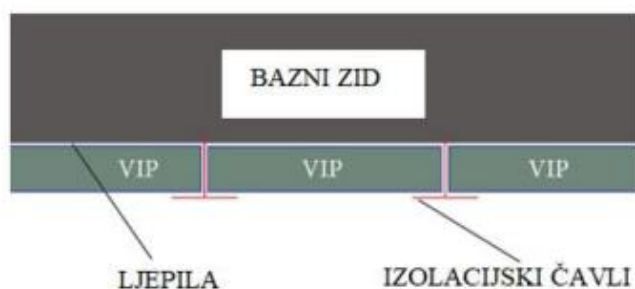
Slika 5.2.2. Shematski prikaz montiranja VIP ploča
