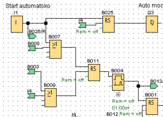
Slika 13 Upravljački dio programa /3 uključivanje timera s kašnjenjem ukapćanja
