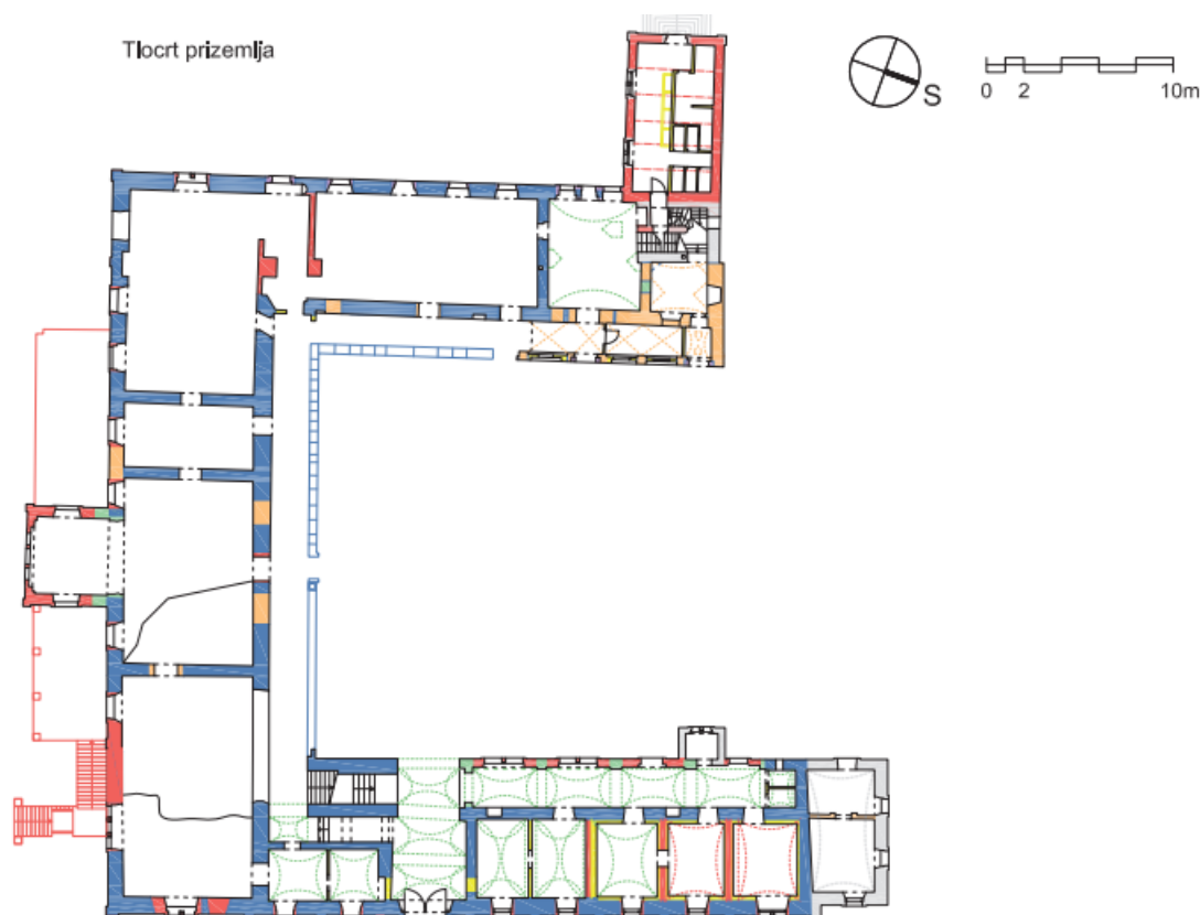
Slika 4. Tlocrt prizemlja dvorca Opeka (Izvor: Puhmajer, 2012)
