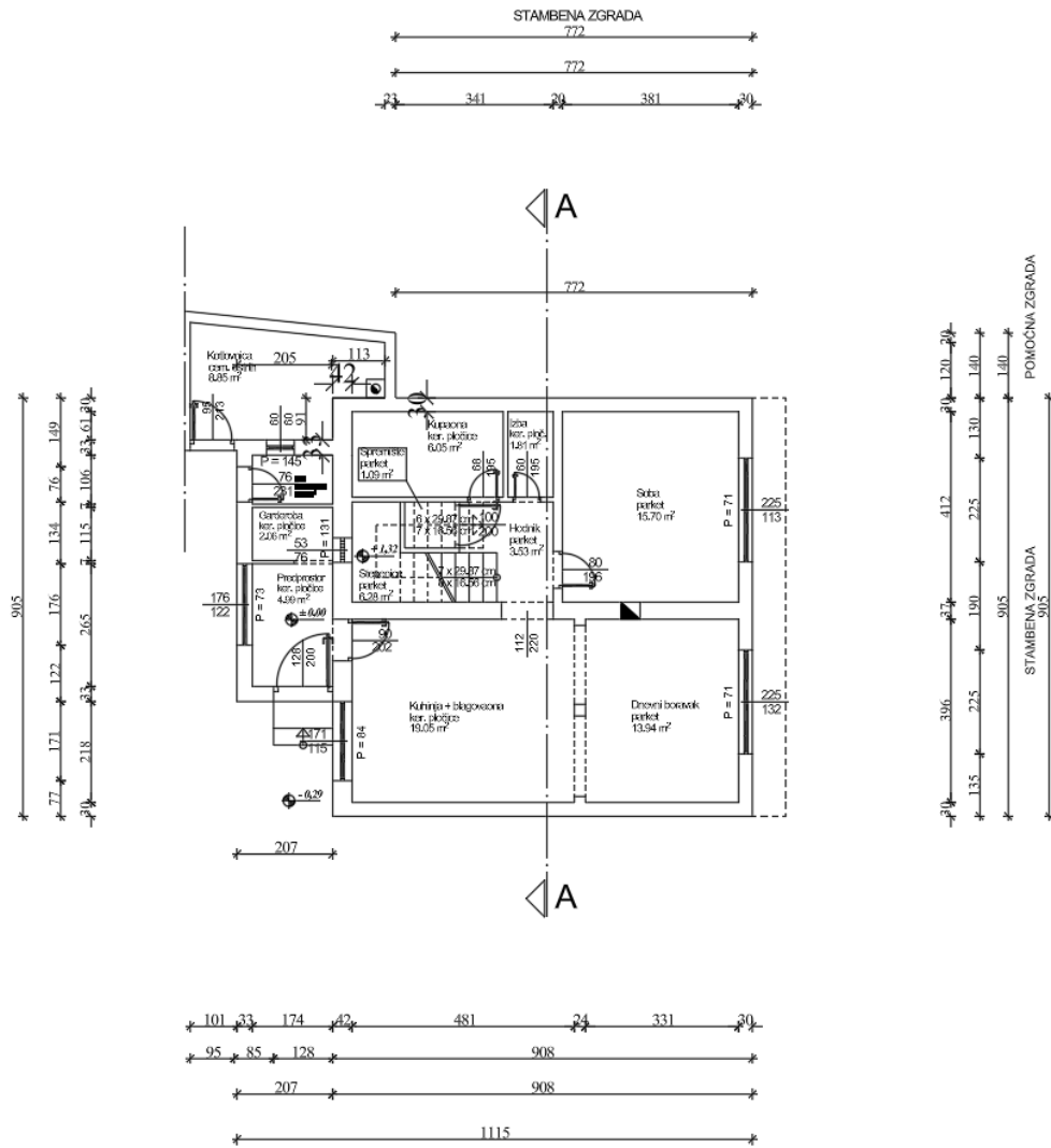
Slika 9 – prizemlje MJ 1:100
