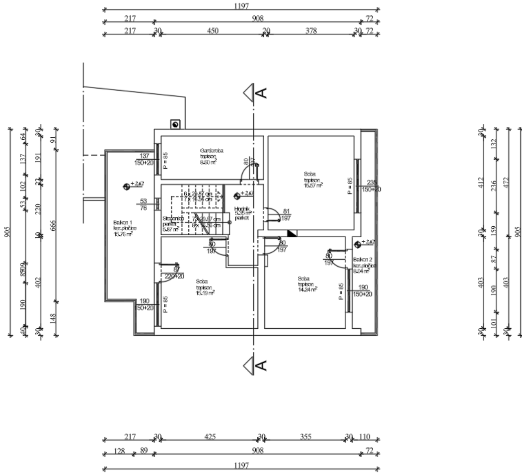
Slika 10 – 1. kat MJ 1:100
