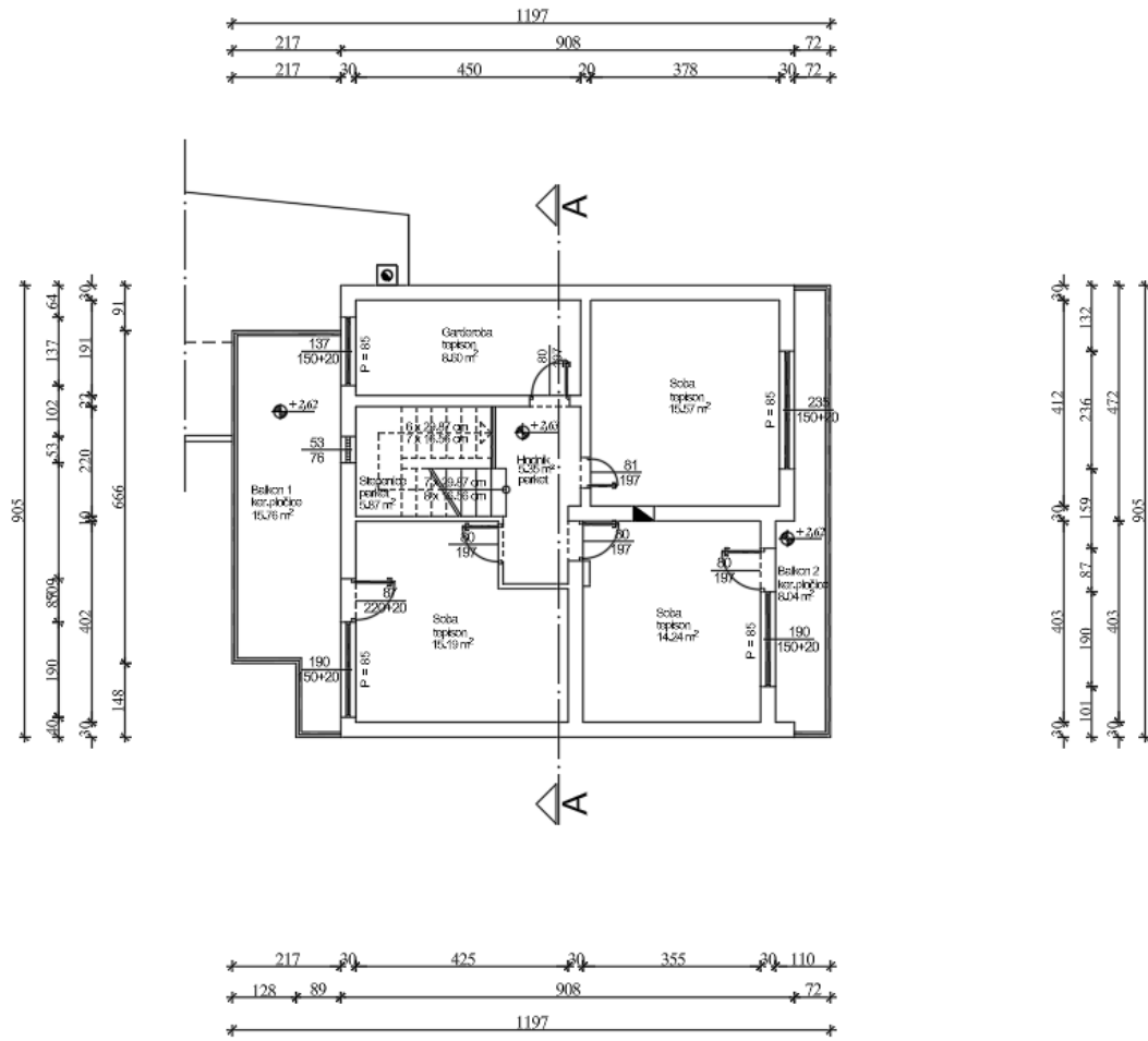
Slika 10 – 1. kat MJ 1:100
