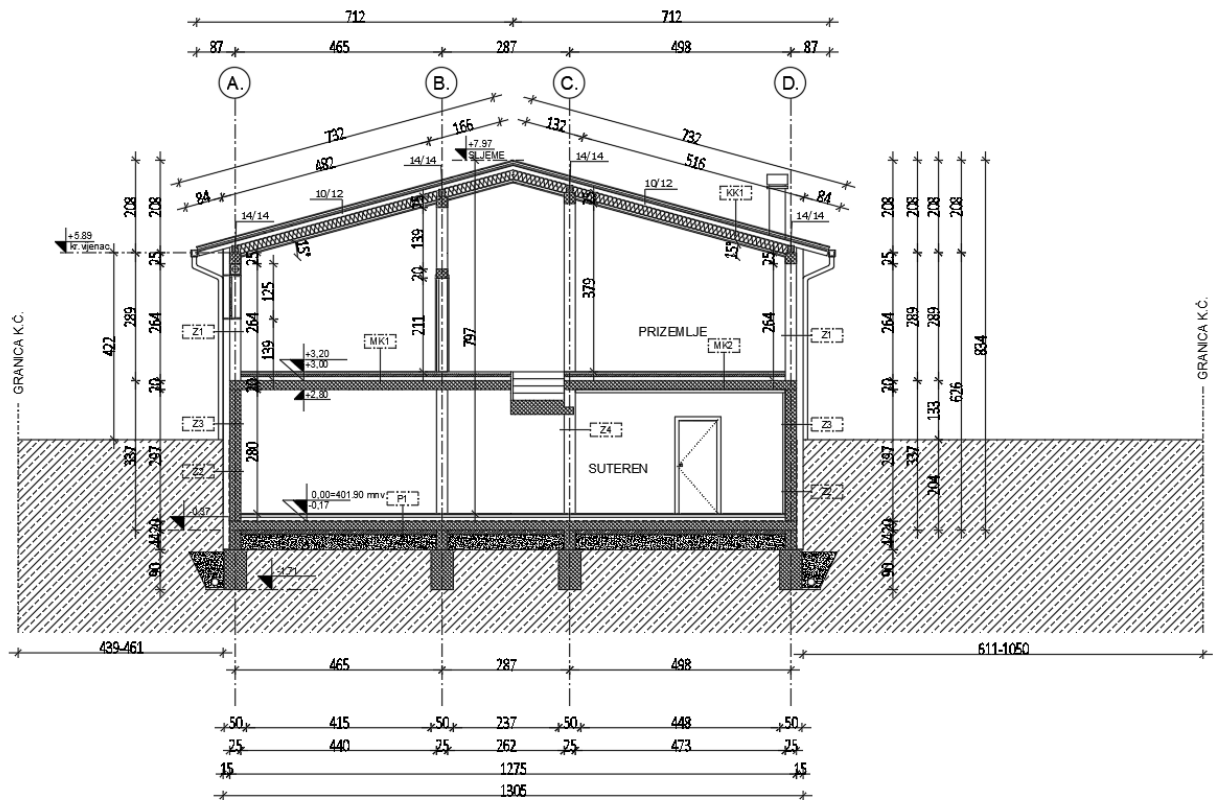
Slika 2.3 Presjek - M 1:100
