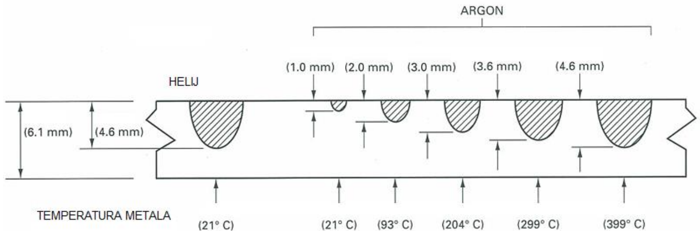
Slika 14 Učinak zaštitnog plina i temperature predgrijavanja na penetraciju zavarenog spoja u bakru TIG zavarivanju s 300 A istosmjernje struje pri brzini zavarivanja od (3-4 mm/s) [4].
