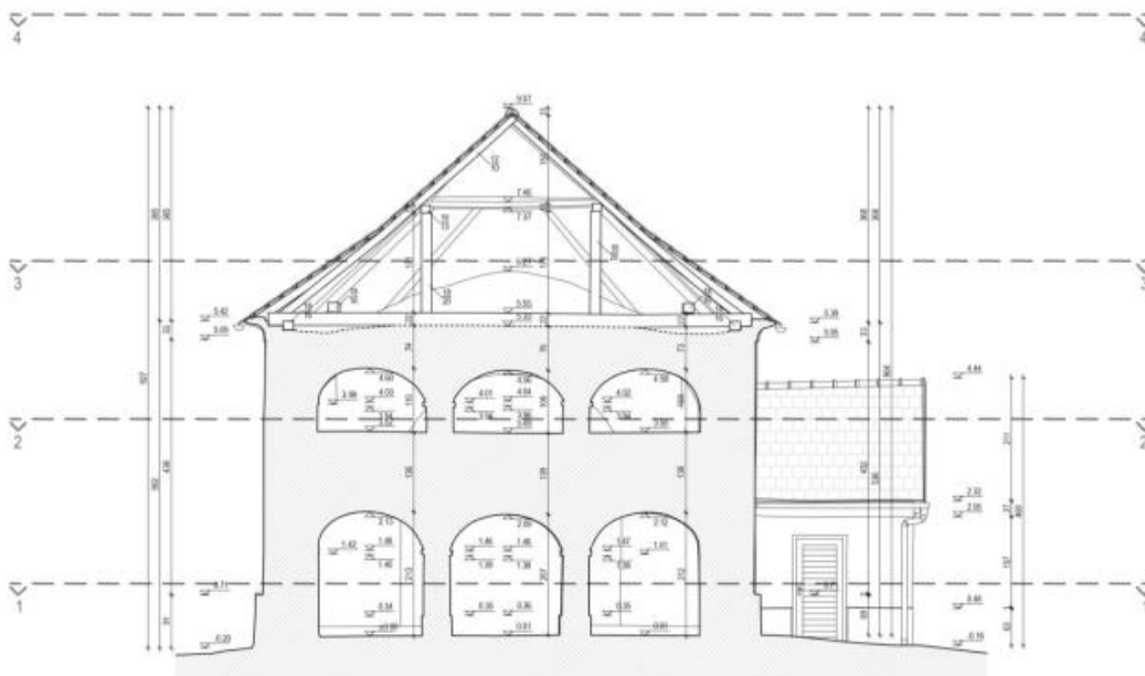
Slika 26: Presjek 3-3 [4]
