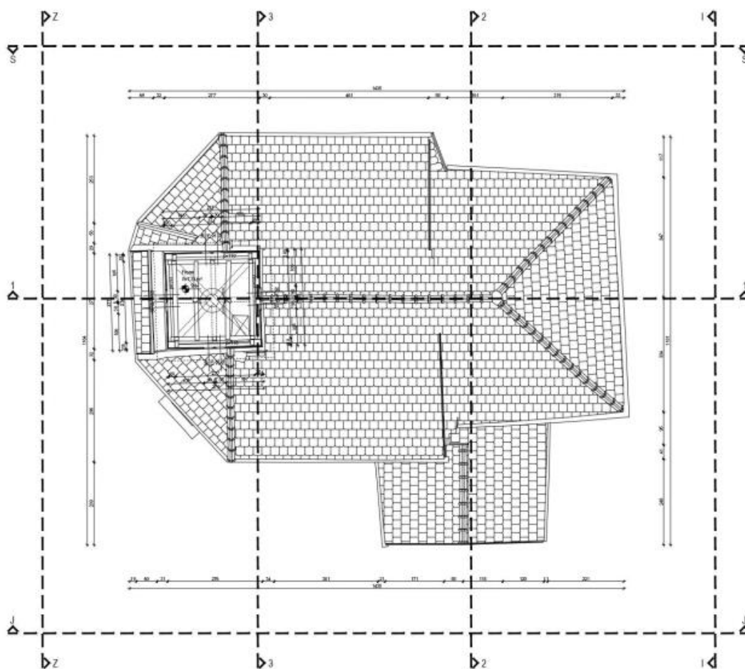
Slika 22: Tlocrt – razina 4 [4]
