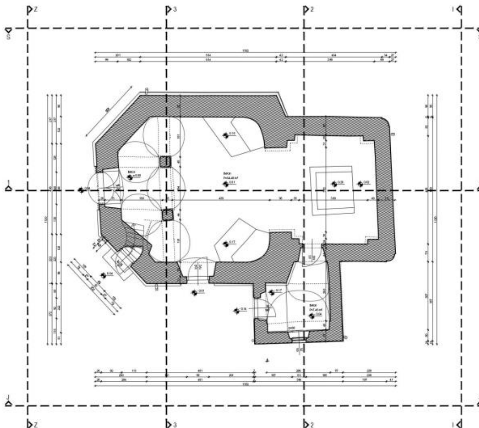
Slika 19: Tlocrt – razina 1[4]
