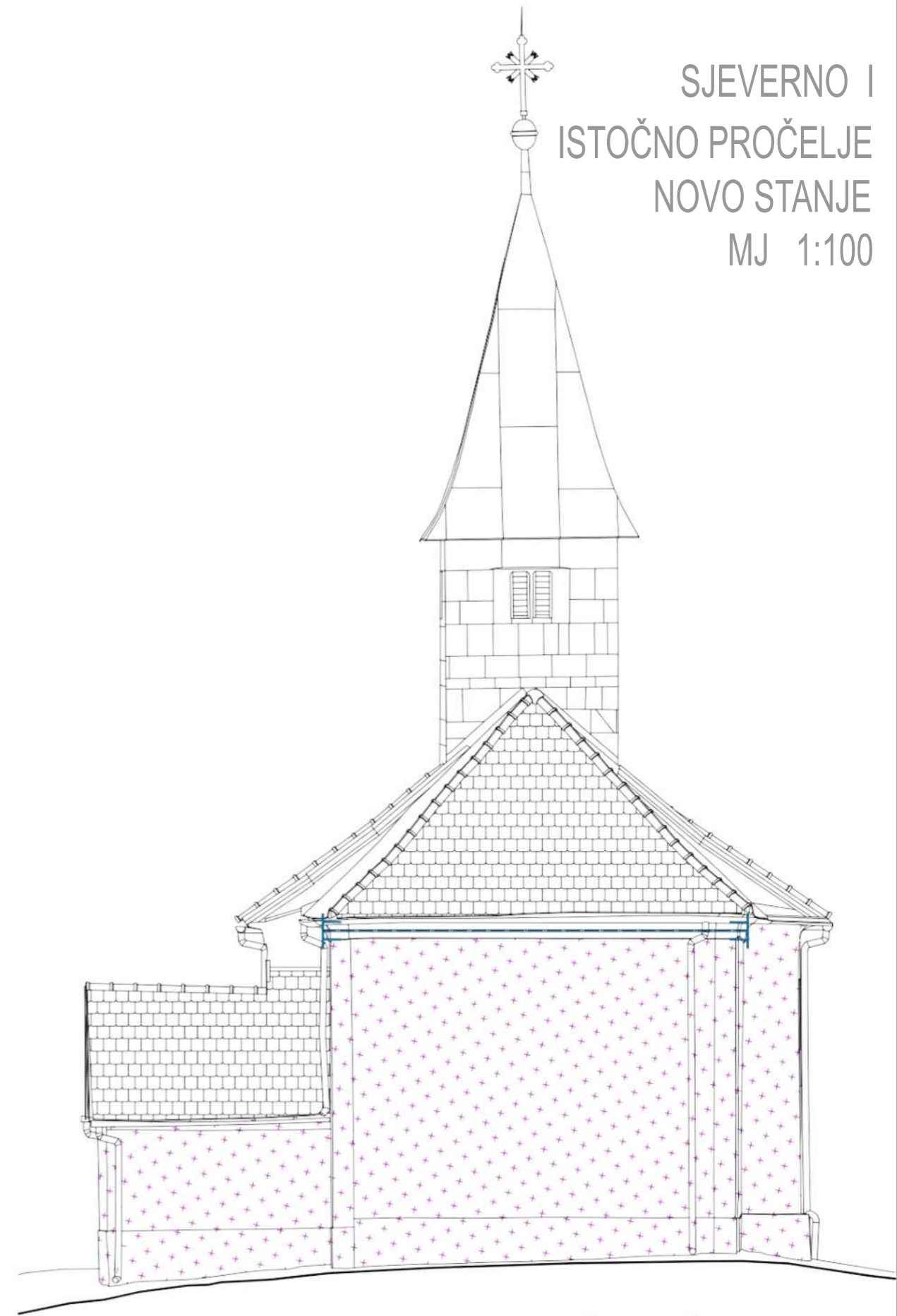
ISTOČNO PROČELJE
