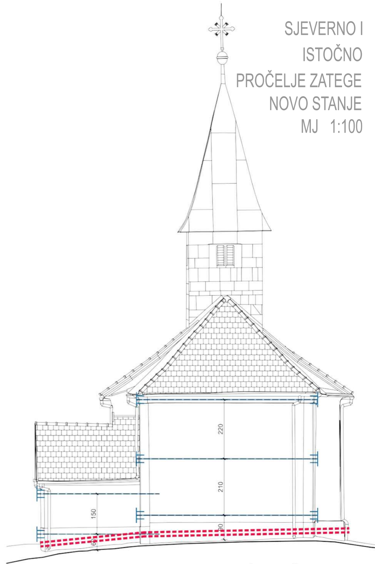
ISTOČNO PROČELJE
