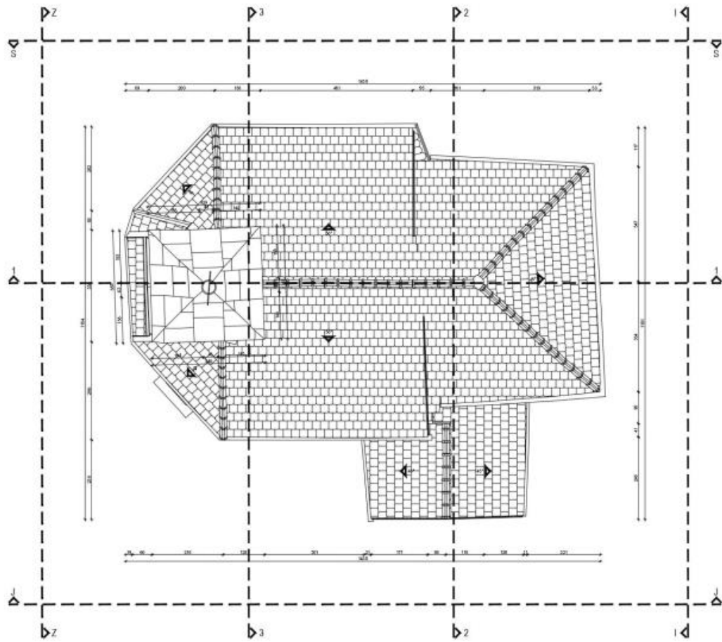
Slika 23: Tlocrt – razina 5 [4]
