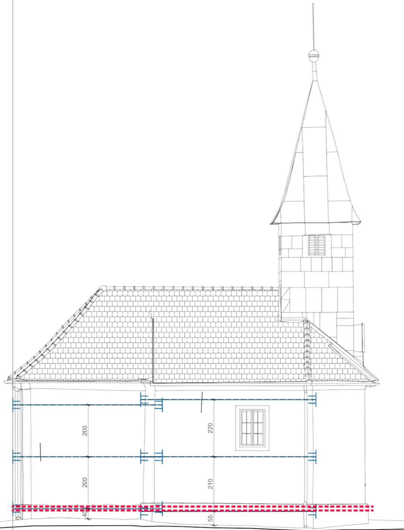
SJEVERNO PROČELJE
