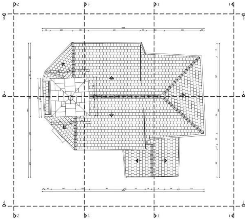
Slika 23: Tlocrt – razina 5 [4]
