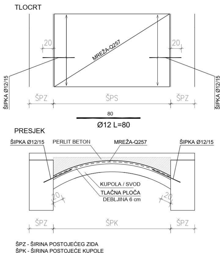
Slika 64: Primjer i prikaz sanacije svoda između zidova [7]
