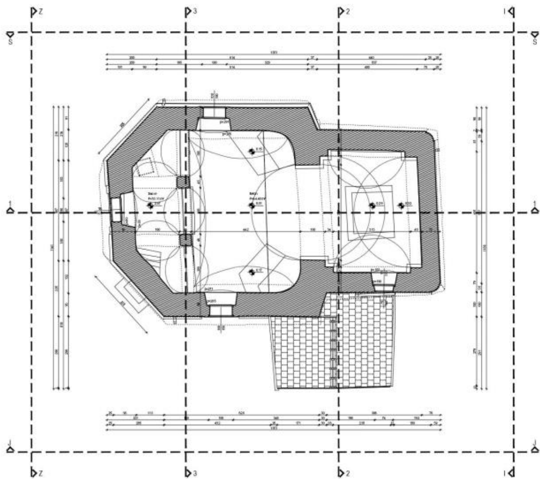
Slika 20: Tlocrt – razina 2 [4]
