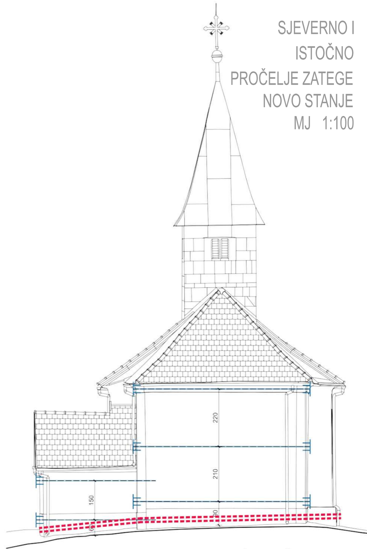
ISTOČNO PROČELJE
