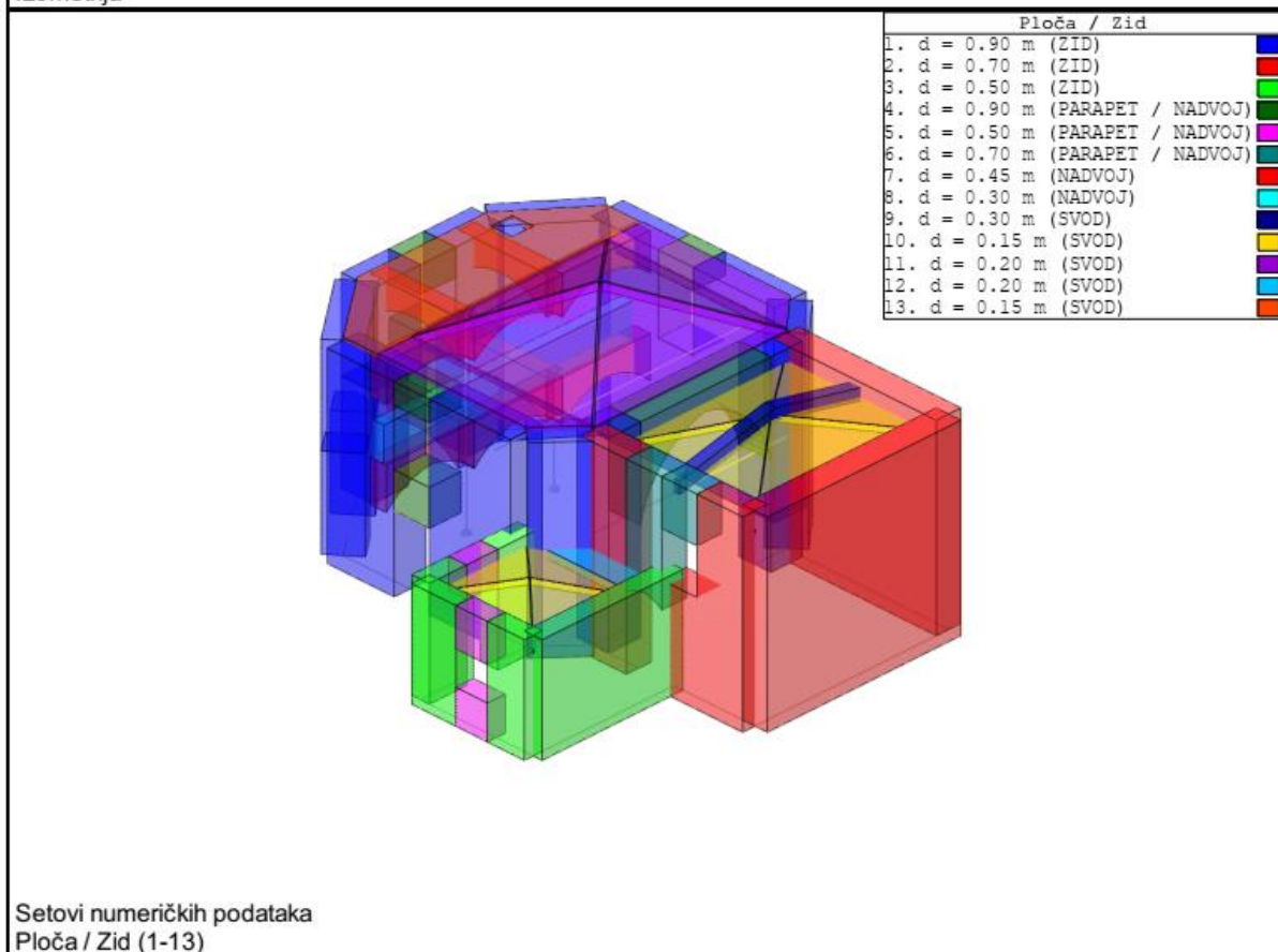
Izometrija
