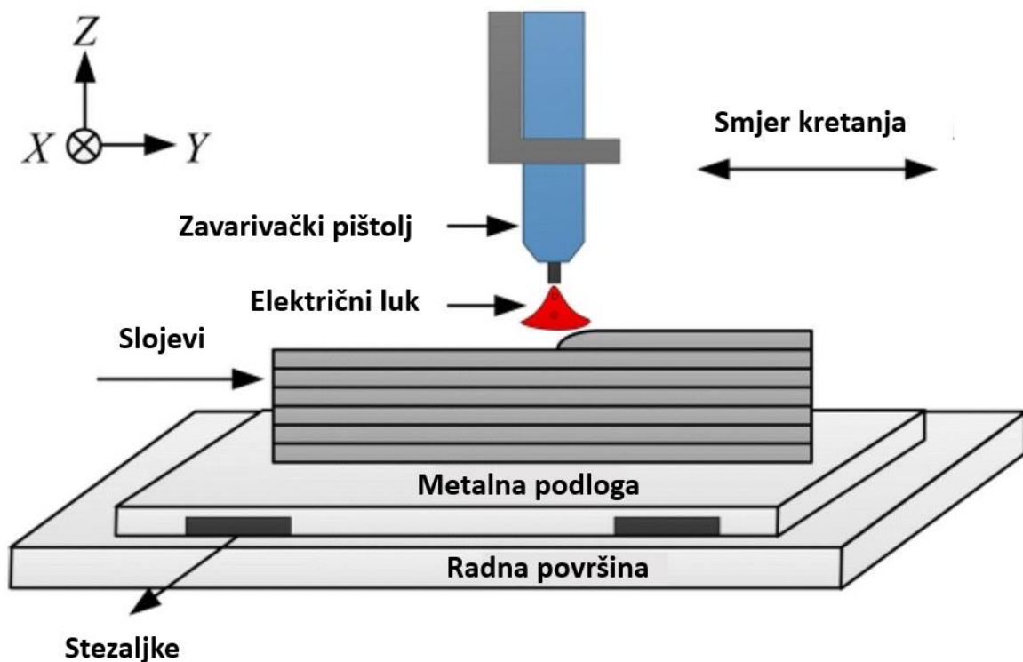
Slika 12: WAAM postupak [16]
