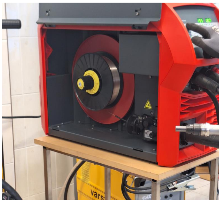
Slika 24: Bočni pogled na uređaj za zavarivanje
