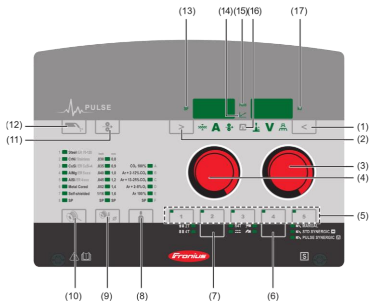
Slika 25: Korisničko sučelje Fronius TransSteel 3000 Puls/FSC uređaja [32]
