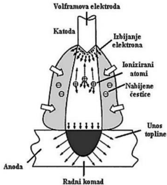
Slika 17. Mehanizam suženja električnog luka [30]
