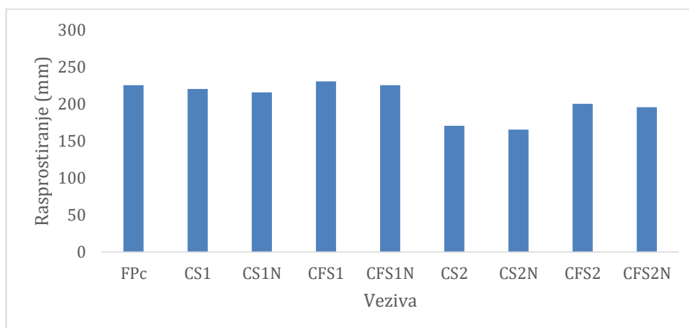
Slika 20. Obradivost geopolimernog veziva [14]
