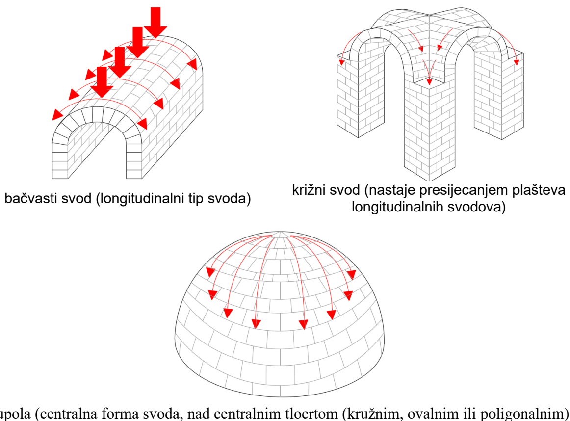
Slika 63. Različiti tipovi svodova sa prikazom prijenosa opterećenja
