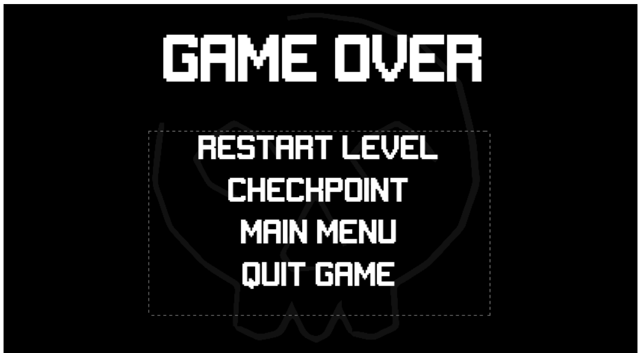
Slika 5.48 Death menu
