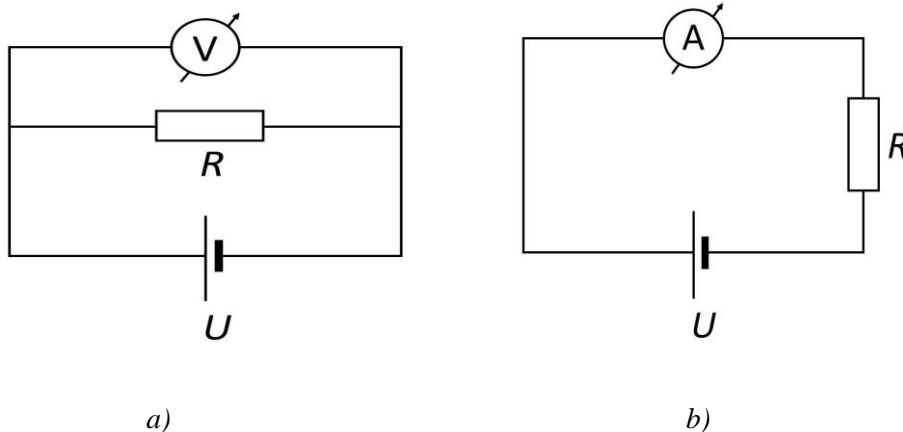
Slika 3.1 Spajanje voltmetra a) i ampermetra b)[10]
