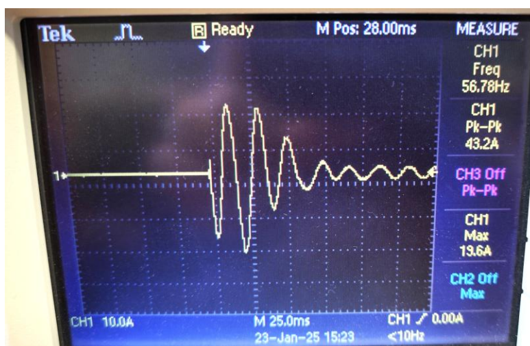
Slika 5.4 Osciloskopski prikaz struje zaleta kod direktnog pokretanja
