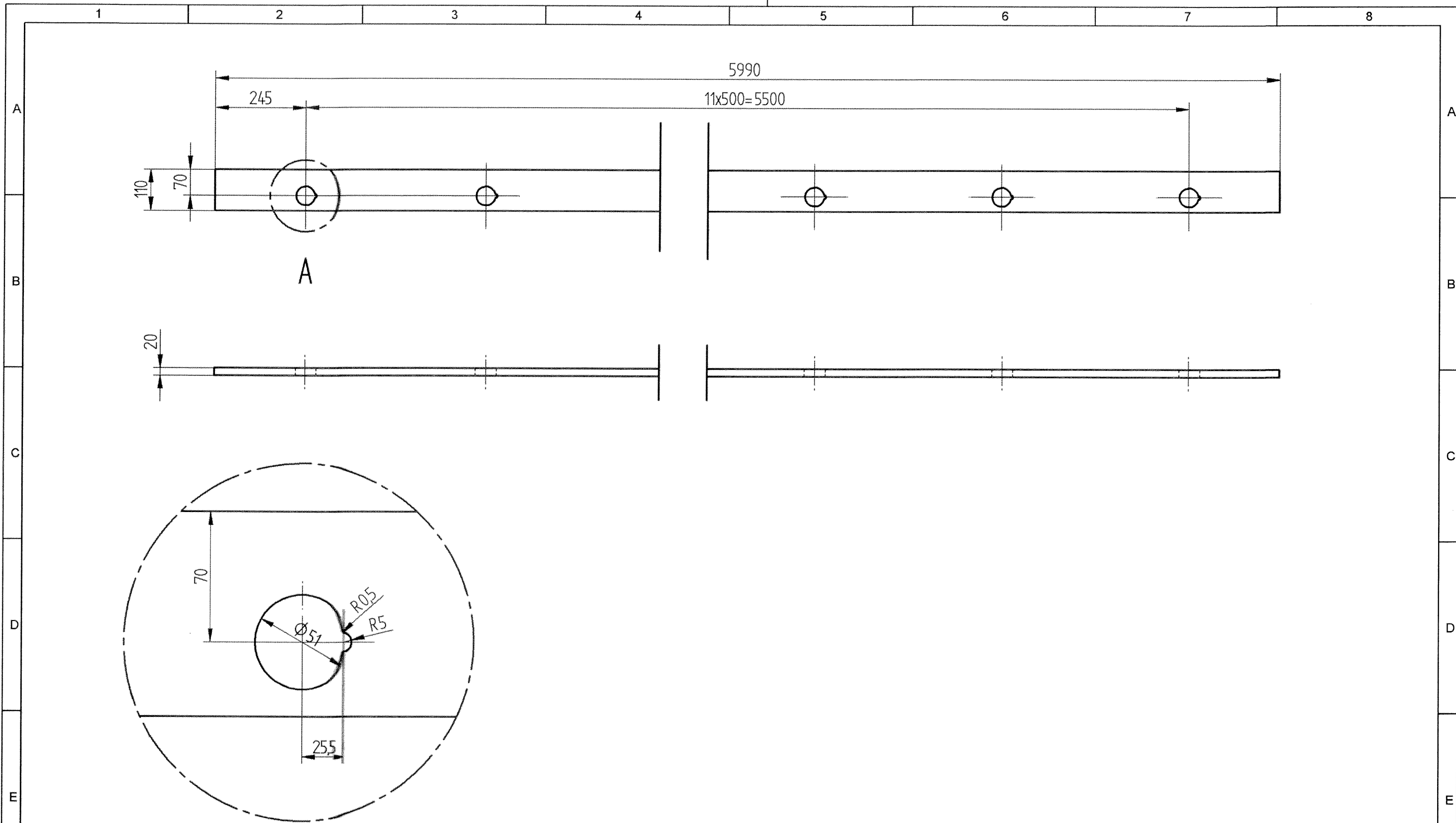
EINZELHEIT A 1:2
