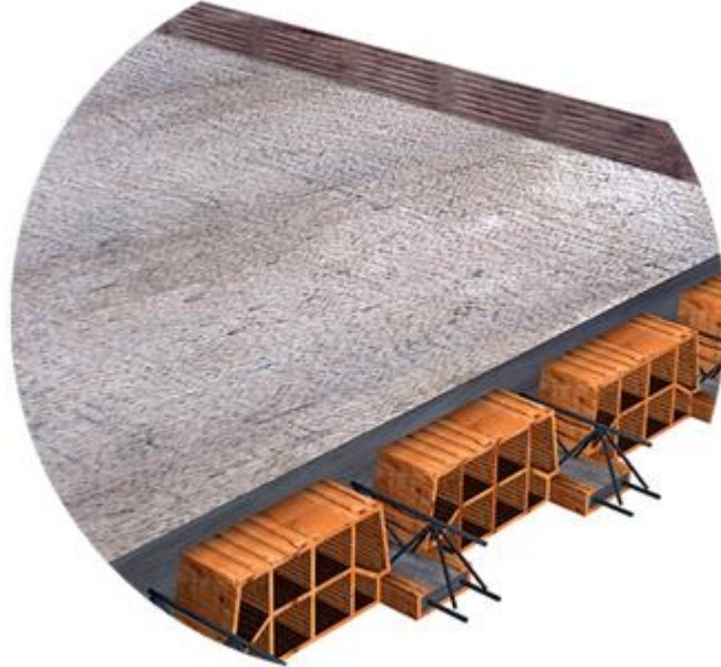
Slika 5.4.1. Rubne trake od kamene vune po obodu zida
