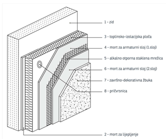
Slika 2.11 ETICS sustav
