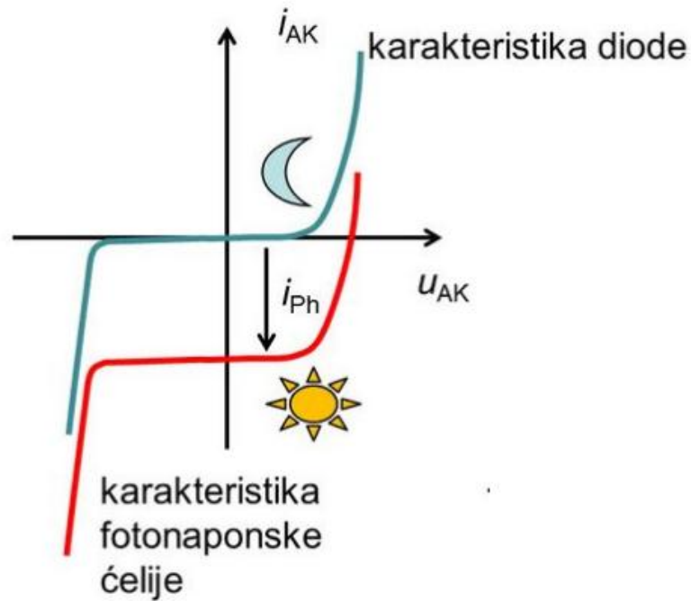
Slika 3.3. Karakteristika solarne ćelije [6]
