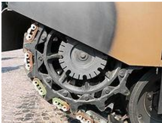
Slika 2.5 Pogonski lančanik od Leclerc glavnog tenka (2006).
