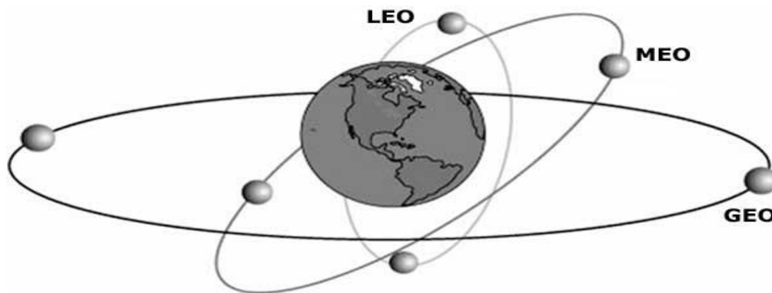
Slika 2.3. Satelitske orbite
