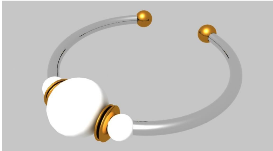
Slika 6.17. Final Gathering
