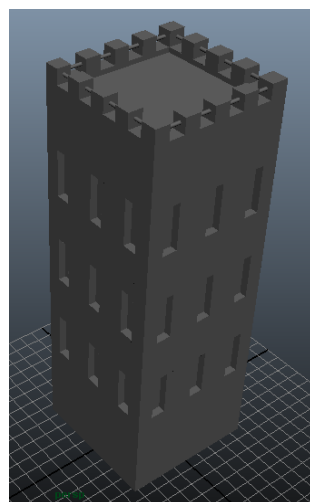
Slika 7.7. Stvoreni prozori
