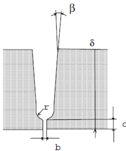
"U" žlijeb
