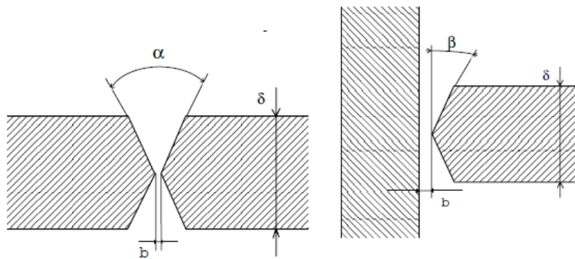
"X" žlijeb
