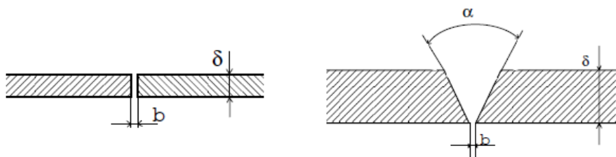
"I" žlijeb
