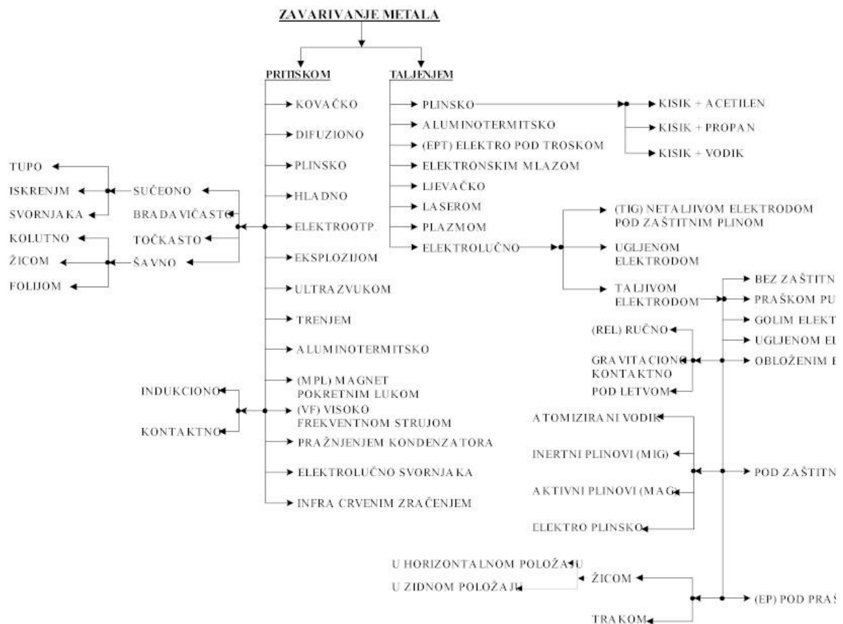
Slika 2.1. Podjela postupa zavarivanja [2]
