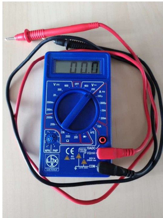
Slika 3.4 Digitalni multimetar
