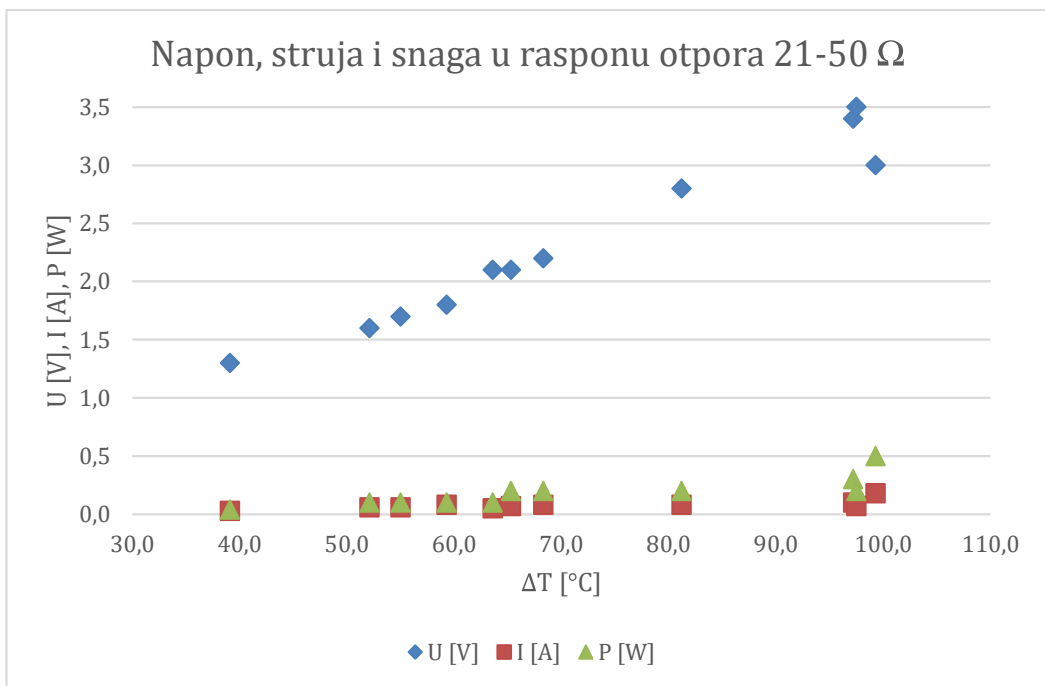
Slika 3.17 Raspon napona od 21 do 50 [ \Omega ]
