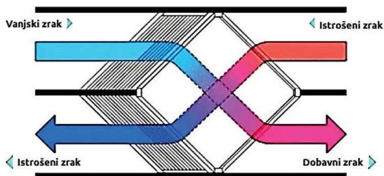
Slika 3.2.1. Pločasti rekuperator – sustav povrata osjetne topline
