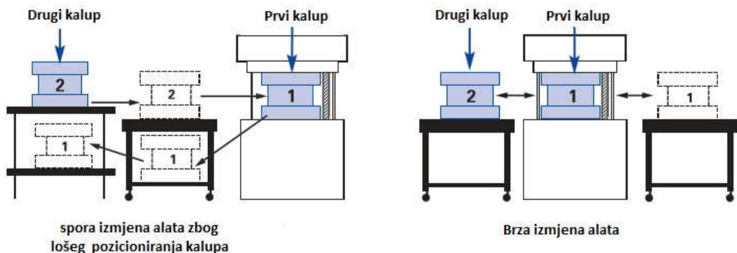
Slika 3.2.1.18.1 Primjer brze izmjene alata primjenom SMED metode [8]
