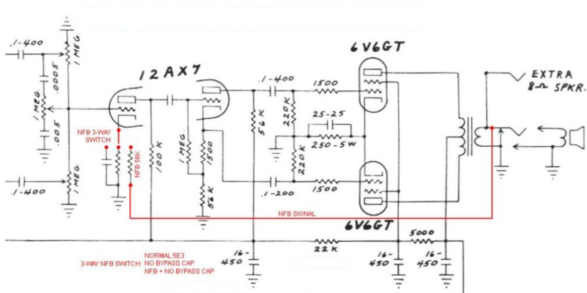
Slika 3.11. Shema spoja; Otpornik od 56\text{k}\Omega je za zvučnik od 8\Omega . Zamjenom s manjom vrijednosti dobiva se veća količina povratne veze. [7]
