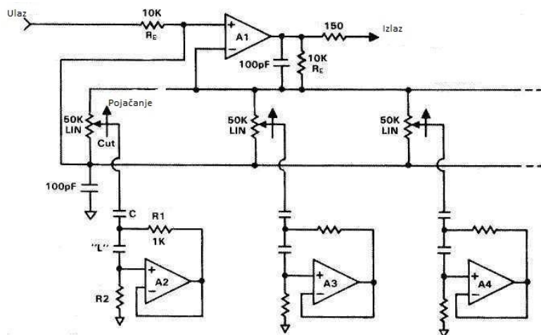
Slika 3.18. Shema spoja [10]
