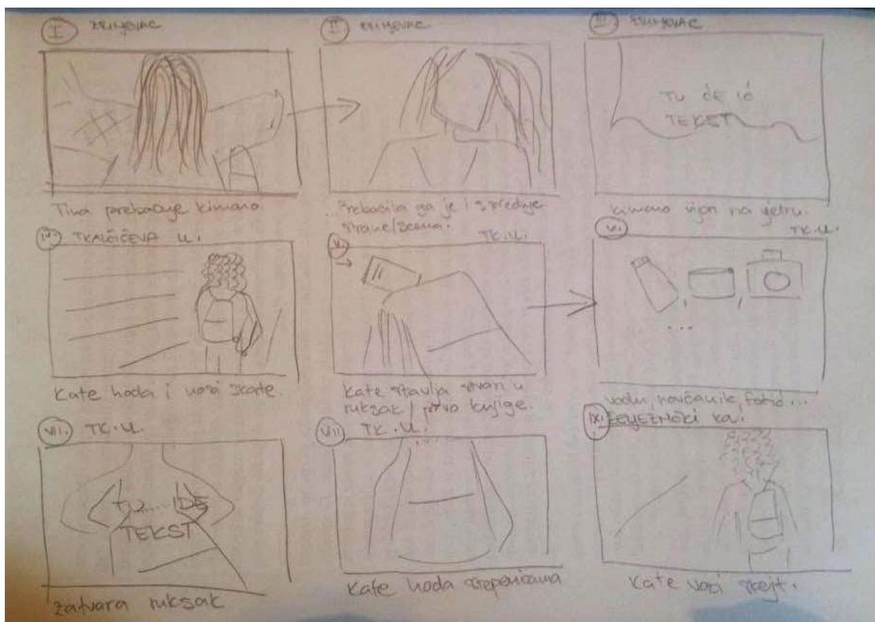
Slika 6.1. Storyboard 1
