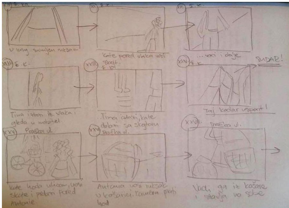
Slika 6.3. Storyboard 3
