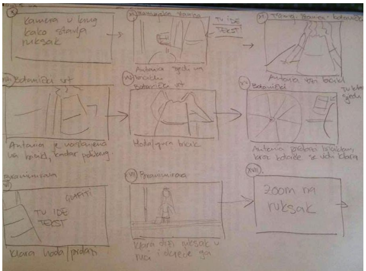
Slika 6.2. Storyboard 2
