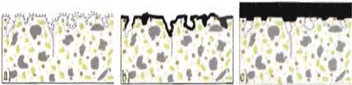
Slika 4.11. Vrste površinske zaštite: a) impregnacija, b) hidrofobna impregnacija, c) premaz
