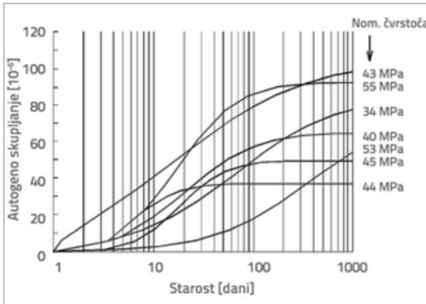
Slika 3.6. Autogeno skupljanje običnih betona
