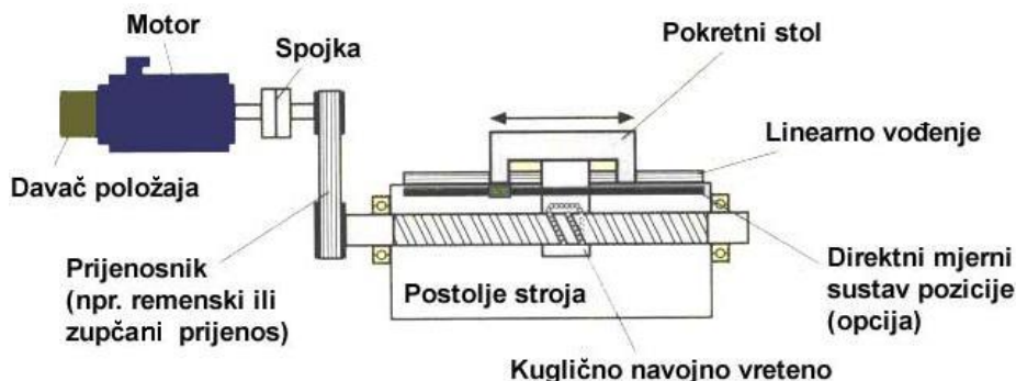
Slika 7.9: Posmični prigon CNC strojeva [19]
