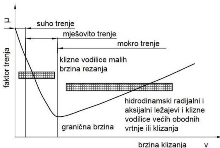
Slika 7.26: Stribeck krivulja [20]
