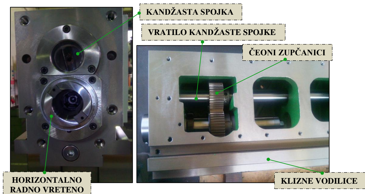
Slika 7.19 : Vretenište CNC glodalice
