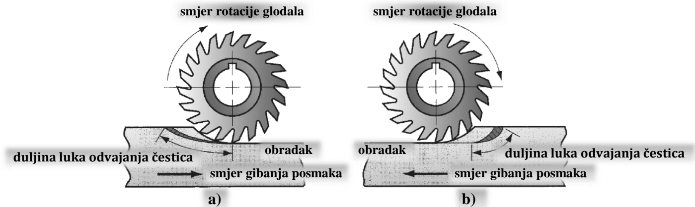
Slika 5.10: Protusmjerni i istosmjerni smjer glodanja
