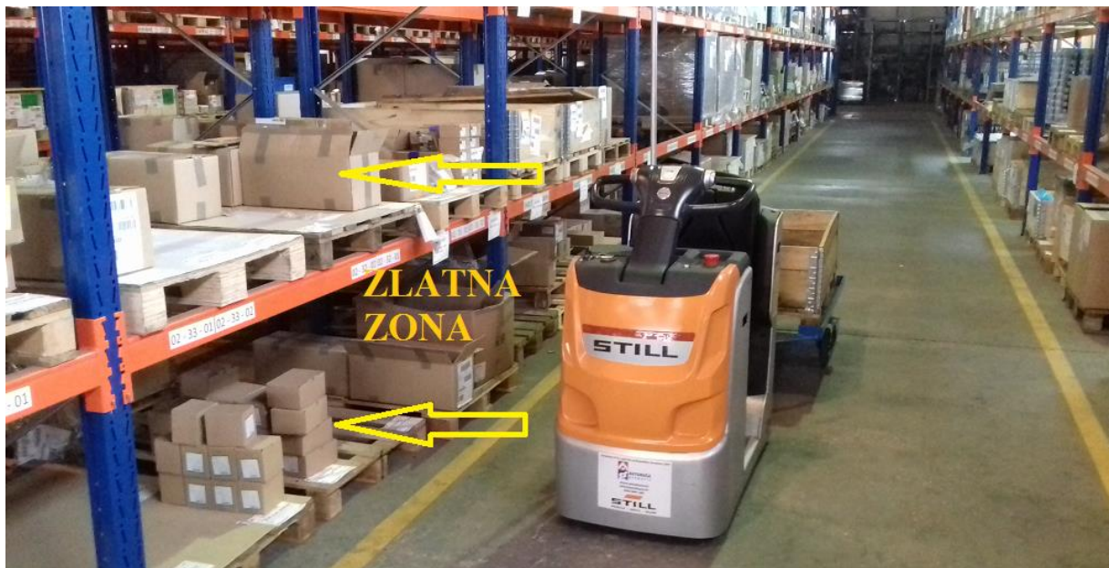
Slika 3.18. Vučno vozilo na lokaciji supermarket skladišta „zlatna zona“ [28]
