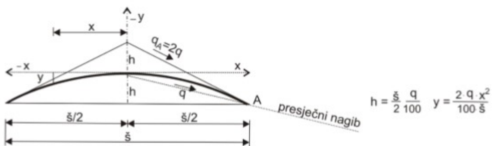
Slika 6.5 Dvostrani parabolični nagib prometnice
