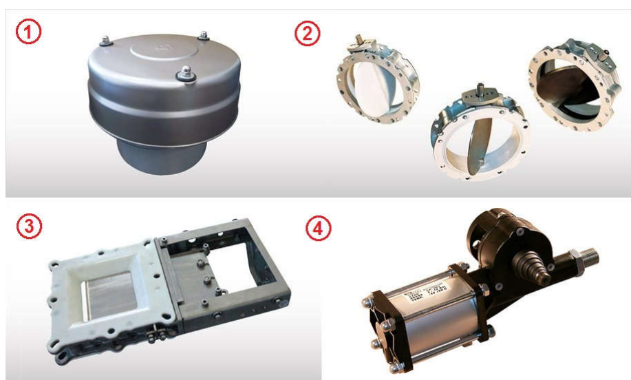
Slika 3.3 Ventil za regulaciju pritiska VCP (1), leptirasti ventil VFS (2), ventil s pomičnim zasunom VIB (3), elektropneumatski pogon CP (4) [26]
