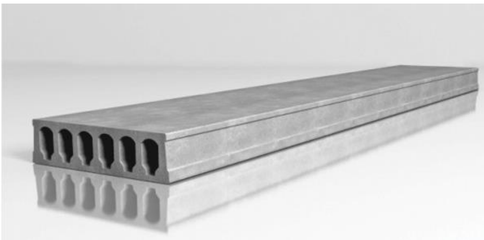
Slika 2.1.1. - Šuplja betonska ploča sistema Širbegović
