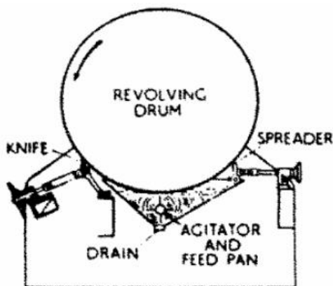
Slika 3.5 Valjkasta sušara [3]
