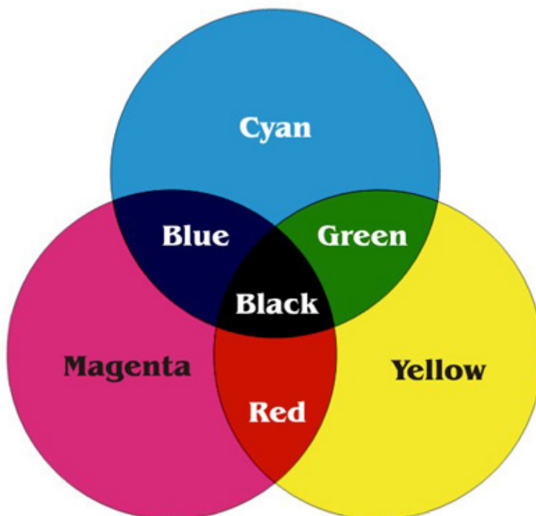
Slika 3.2. Suptraktivna sinteza
