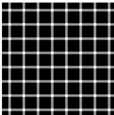
Slika 6.15. Hermanova iluzija
