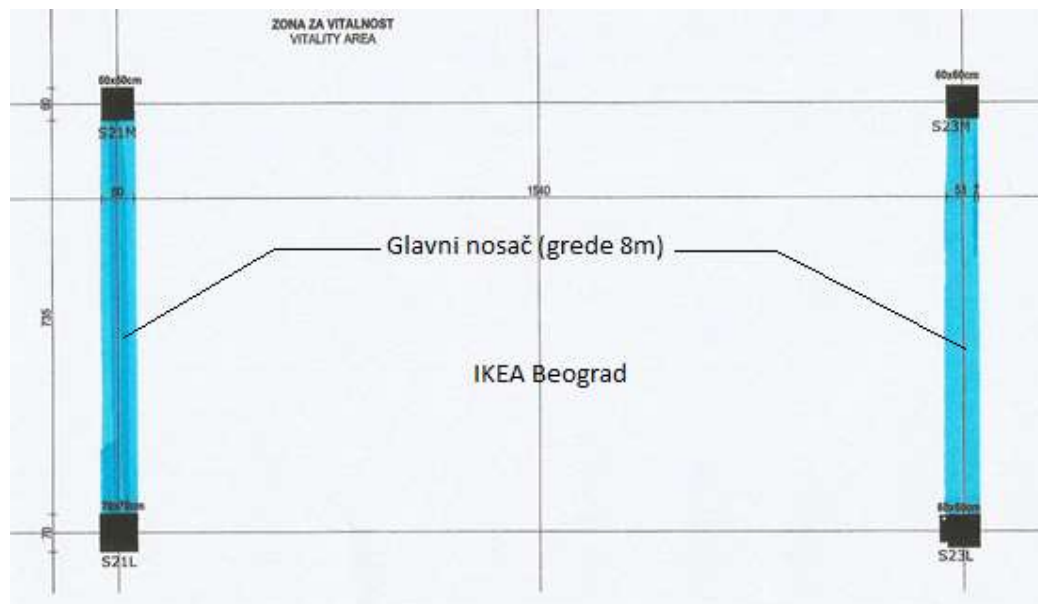
Slika 6.11. Tlocrt oslanjanja prednapregnute grede na stupove - IKEA
