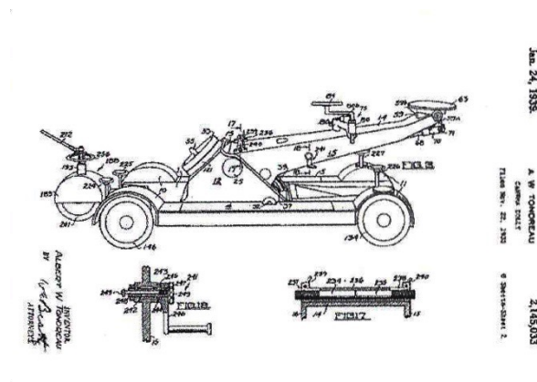
Slika 3-4 Warner Bros camera dolly 1935. [2]
