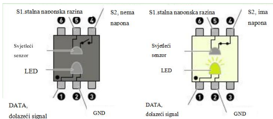
Slika 5.2 Optokapler [16]
