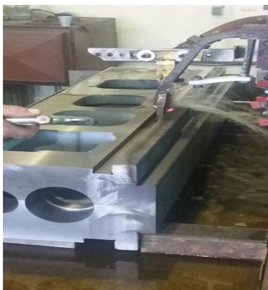
Slika 25. Indukcijsko kaljenje vodilica
