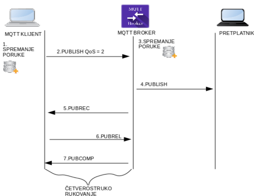
Slika 5.2 Primjer komunikacije koristeći najvišu kvalitetu usluge (QoS 2)
