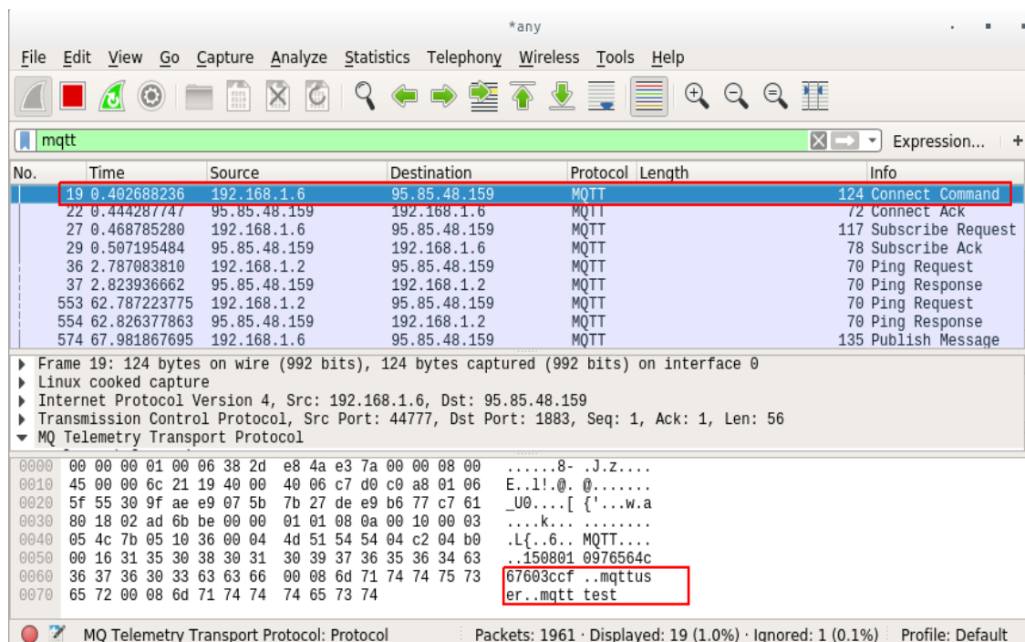
Slika 6.23 Prikaz sadržaja zarobljenog CONNECT MQTT paketa is kojega se može pročitati korisničko ime i lozinka
