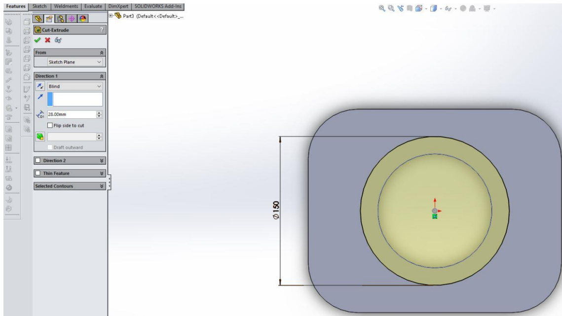
Slika 4.3 Četvrti korak modeliranja (rupa \text{\O}150 mm) [10]
