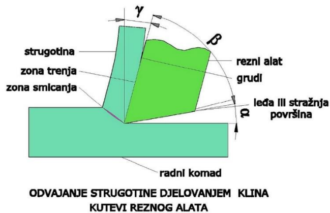
Slika 2.1 Osnovni postupak strojne obrade odvajanjem estica [2]
