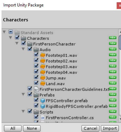
Slika 7.35 Character prozor
