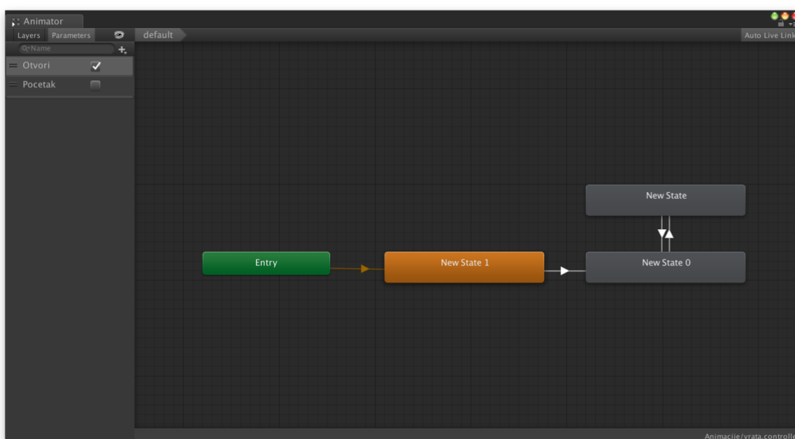
Slika 5.9. Animator View
