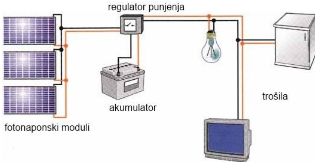
Slika 1.1 Dijelovi otočnog sustava [3]
