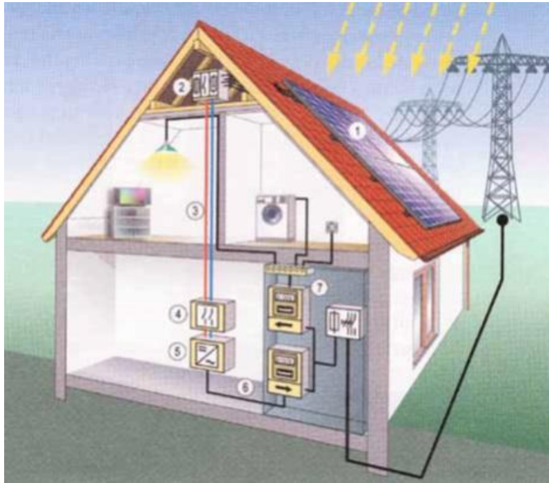
Slika 4. Fotonaponski sustav priključen na javnu mrežu preko kućne instalacije [5]
