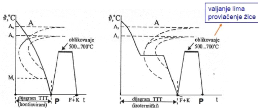
Dijagram 5. Perliforming postupak [16]
