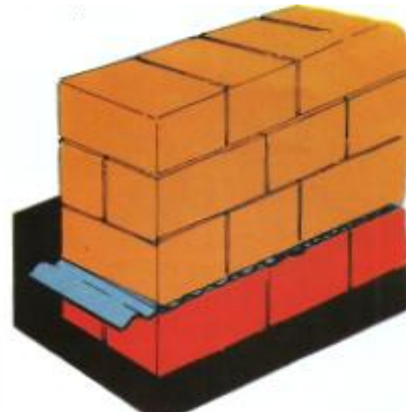
Slika 35. Postavljanje nehrđajućeg valovitog lima u rešku između redova opeka
