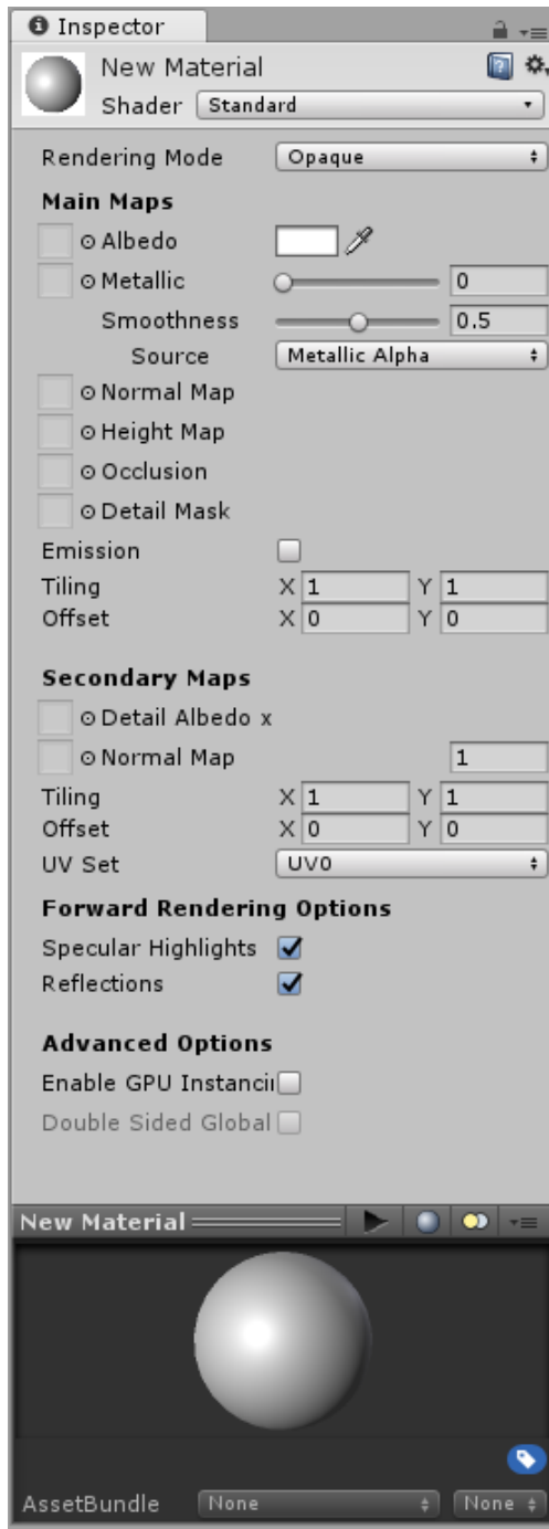
Slika 4.4. Standardni shader
