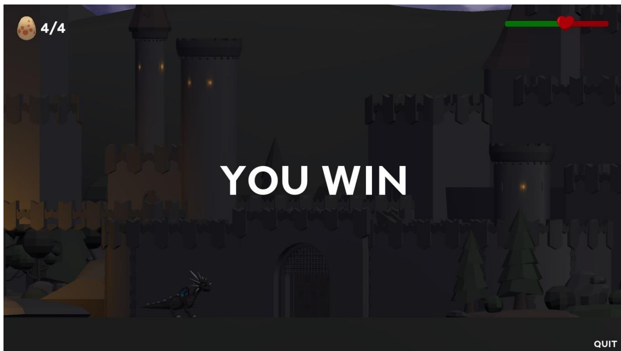
Slika 6.76. Igra Dexter 4
