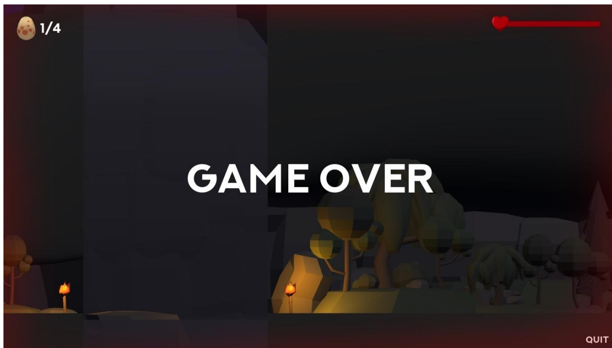
Slika 6.75. Igra Dexter 3
