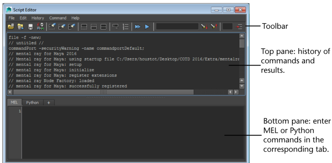
Slika 3.32. Script Editor [18]
