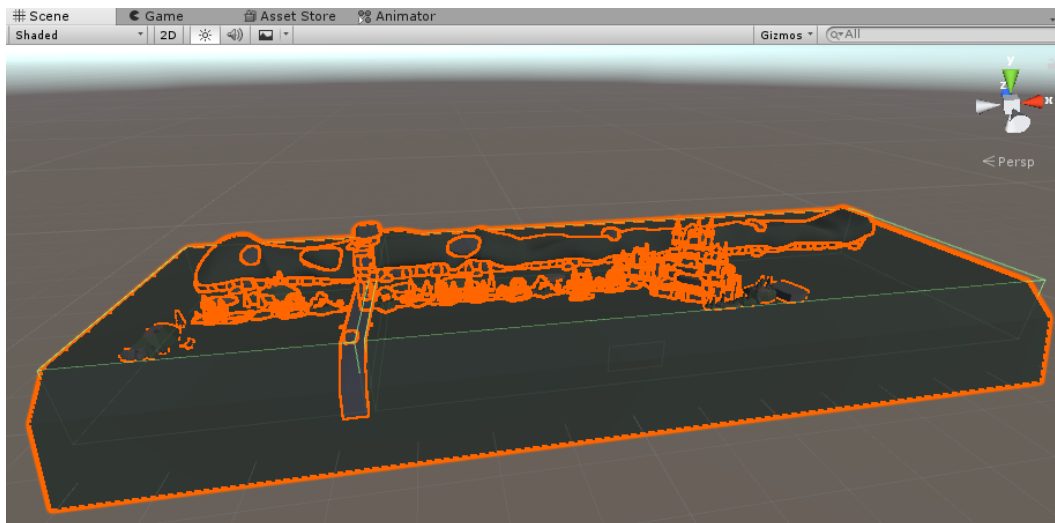
Slika 6.21. Updateana scena
