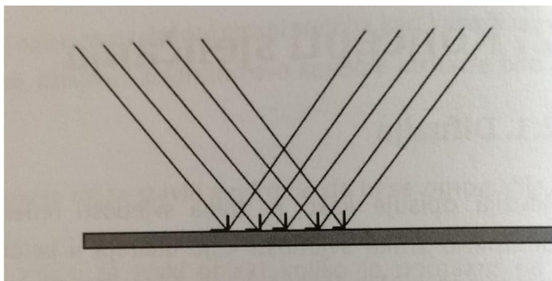
Slika 5.2 Refleksija [19]
