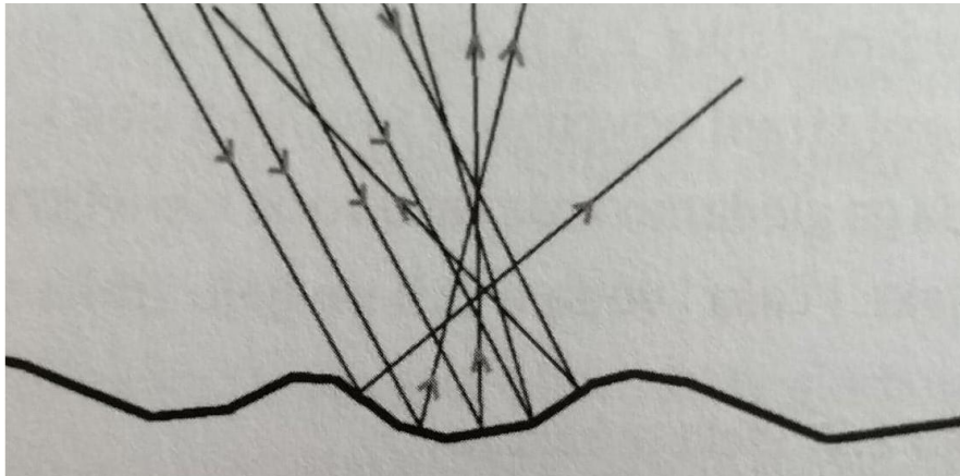
Slika 5.1 Difuzija [18]
